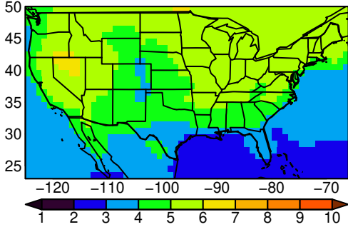
HadGEM3-GC31-LL tasmin SON ssp2
