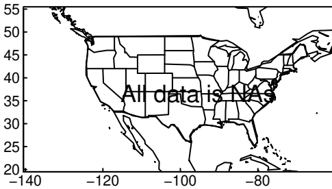
CNRM-CM6-1-HR tasmax SON ssp37
