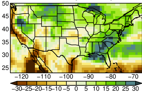
MRI-ESM2-0 pr SON ssp245
