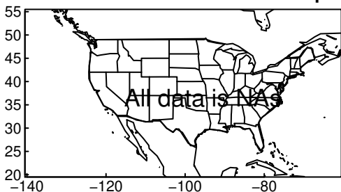
CNRM-CM6-1-HR tasmin MAM ssp24
