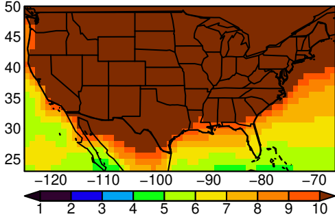
NESM3 tasmin SON ssp245
