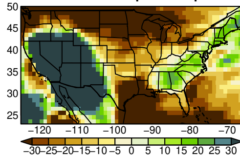
UKESM1-0-LL pr SON ssp585
