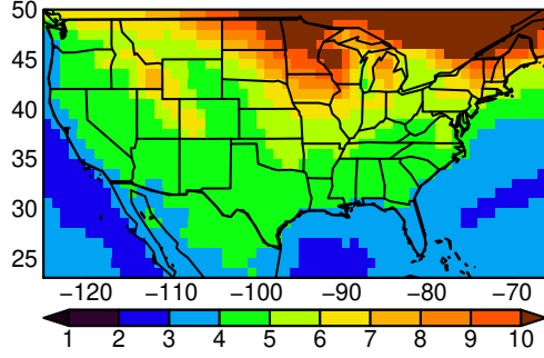
IPSL-CM6A-LR tasmin MAM ssp370
