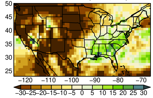
MPI-ESM1-2-HR pr SON ssp585
