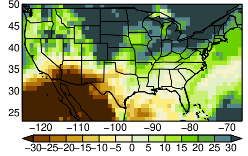
CNRM-CM6-1-HR pr MAM ssp585
