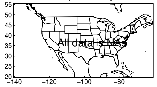
NESM3 pr MAM ssp585
