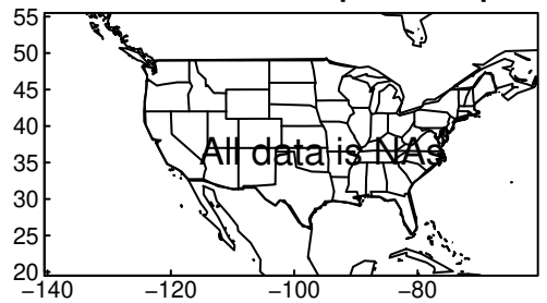
HadGEM3-GC31-MM pr SON ssp585
