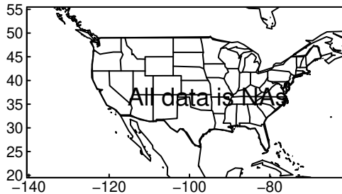
EC-Earth3-Veg pr SON ssp585
