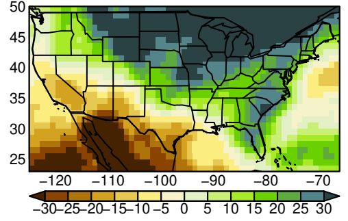
CESM2 pr JJA ssp585
