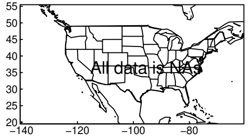
HadGEM3-GC31-MM pr MAM ssp585
