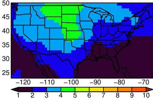
MPI-ESM1-2-LR tasmax SON ssp24f
