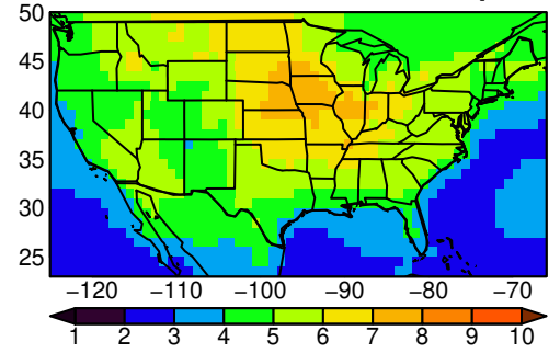
BCC-CSM2-MR tasmin SON ssp585
