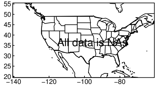
CESM2-FV2 pr MAM ssp585
