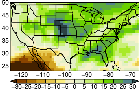
MRI-ESM2-0 pr MAM ssp245
