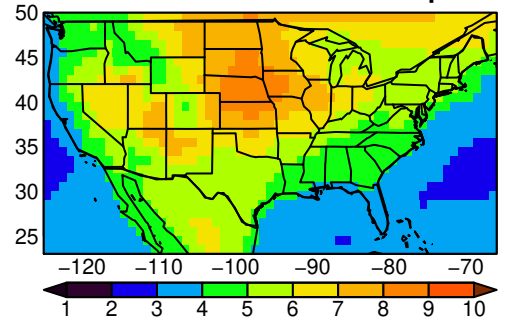
CNRM-CM6-1 tasmx MAM ssp585
