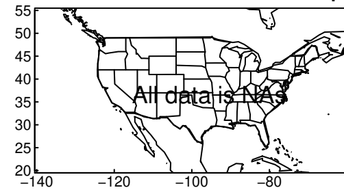
HadGEM3-GC31-MM tasmax SON ssp3
