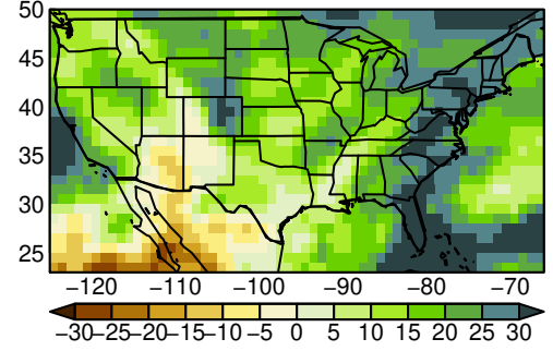
BCC-CSM2-MR pr MAM ssp585
