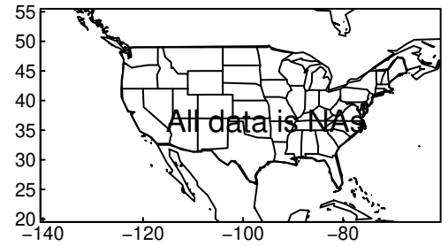
MPI-ESM1-2-LR tasmax SON ssp58f
