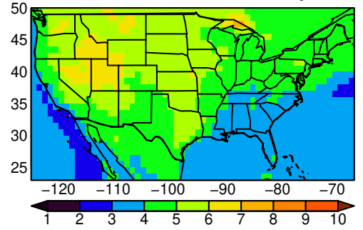
MRI-ESM2-0 tasmax SON ssp585
