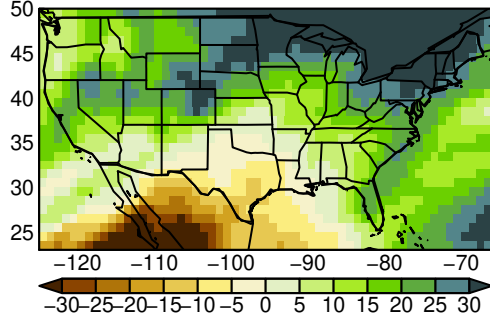
CESM2 pr MAM ssp370
