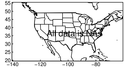
HadGEM3-GC31-MM tasmax MAM ssp5
