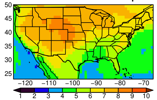
CNRM-CM6-1 tasmx SON ssp585
