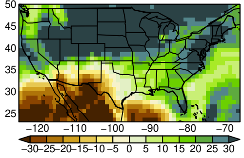
EC-Earth3 pr MAM ssp585
