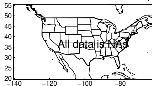
HadGEM3-GC31-MM tasmin SON ssp5
