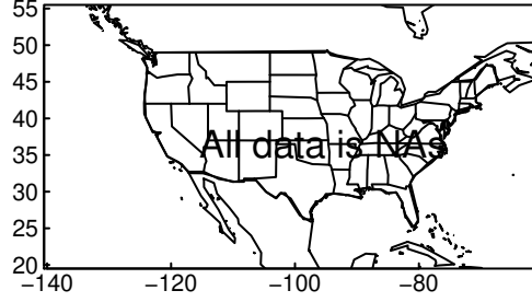
HadGEM3-GC31-LL tasmax MAM ssp3
