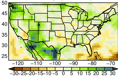
FGOALS-g3 pr SON ssp245
