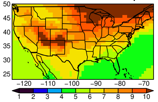
UKESM1-0-LL tasmax MAM ssp585
