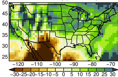
EC-Earth3-Veg pr MAM ssp245
