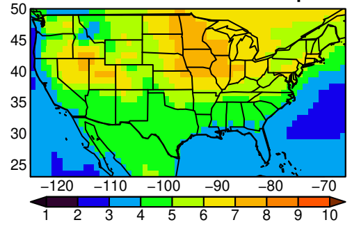
NorESM2-MM tasmx MAM ssp585
