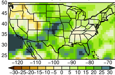
FGOALS-g3 pr MAM ssp245
