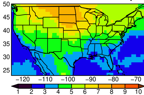
MPI-ESM1-2-HR tasmax SON ssp58i
