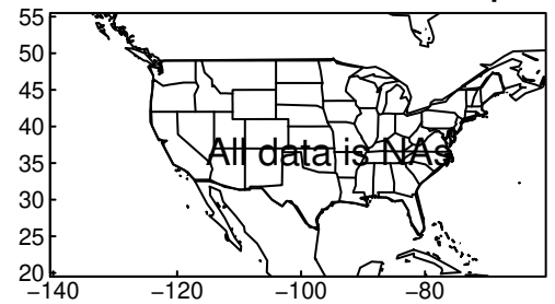
MPI-ESM1-2-LR tasmin SON ssp585
