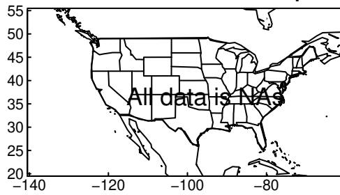
GISS-E2-1-G tasmin SON ssp370
