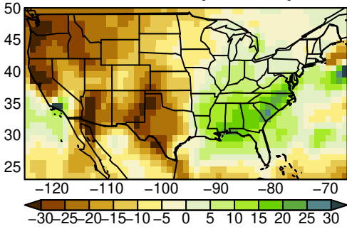
MPI-ESM1-2-LR pr SON ssp245
