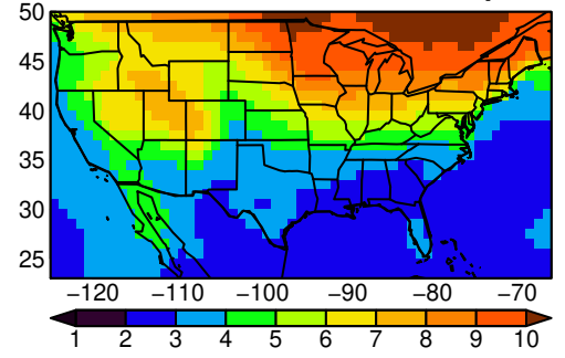
BCC-CSM2-MR tasmin MAM ssp585
