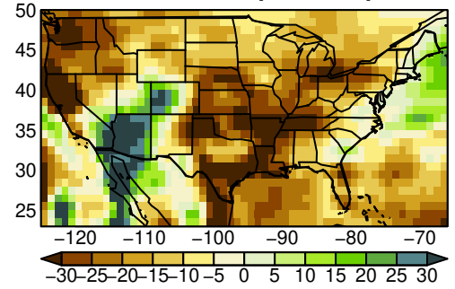
BCC-CSM2-MR pr SON ssp585
