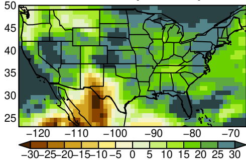
UKESM1-0-LL pr MAM ssp245
