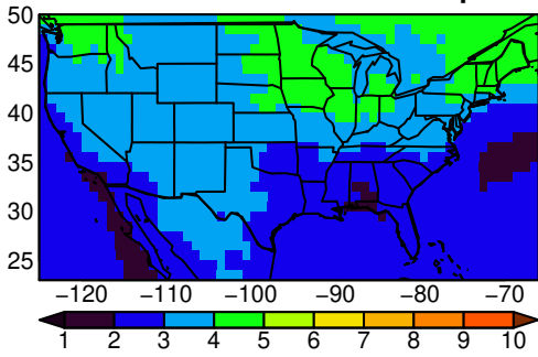
NorESM2-MM tasmx SON ssp245
