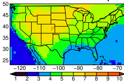
CNRM-CM6-1 tasmx SON ssp370
