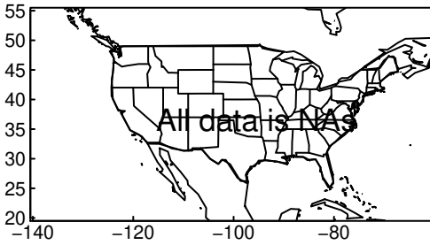
HadGEM3-GC31-MM pr DJF ssp370
