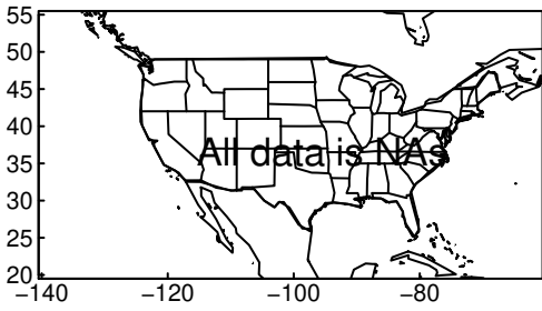
NorCPM1 pr SON ssp245
