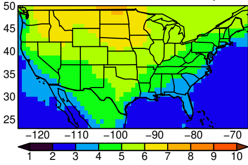
ACCESS-CM2 tasmax SON ssp245
