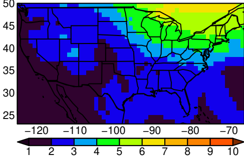
MRI-ESM2-0 tasmin MAM ssp245
