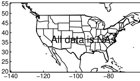
CNRM-CM6-1-HR pr MAM ssp245
