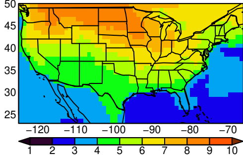
HadGEM3-GC31-LL tasmax SON ssp2
