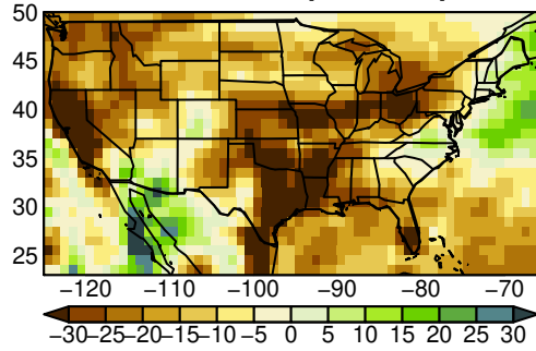
BCC-CSM2-MR pr SON ssp370
