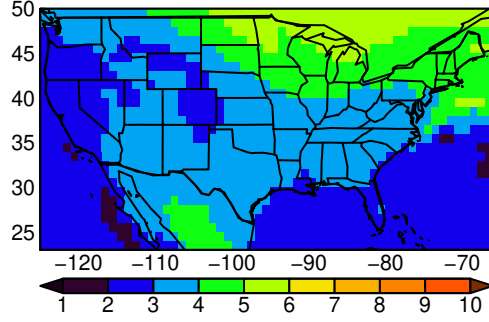
AWI-CM-1-1-MR tasmax MAM ssp37i
