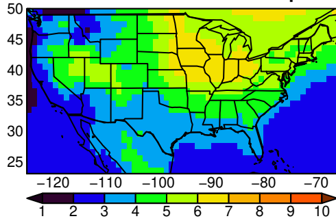
NorESM2-MM tasmx MAM ssp370
