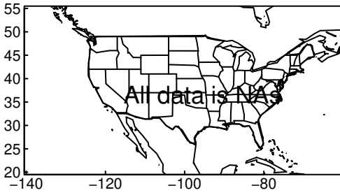
GISS-E2-1-G tasmin DJF ssp245
