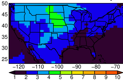
MPI-ESM1-2-HR tasmax SON ssp24i
