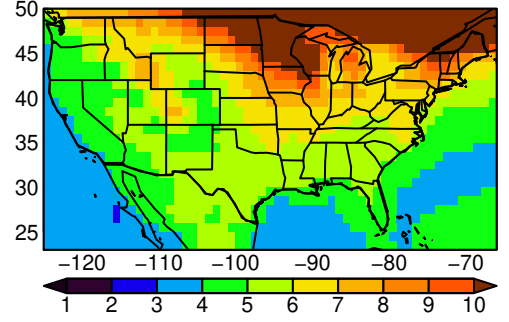
IPSL-CM6A-LR tasmin MAM ssp585
