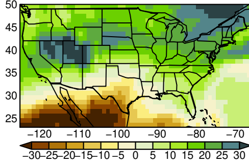
MRI-ESM2-0 pr MAM ssp370
