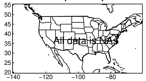
NESM3 pr SON ssp585
