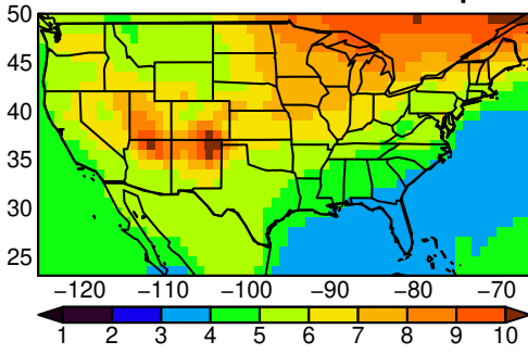
UKESM1-0-LL tasmax MAM ssp370
