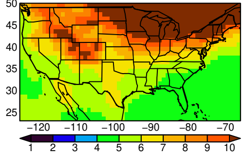
HadGEM3-GC31-LL tasmin MAM ssp5
