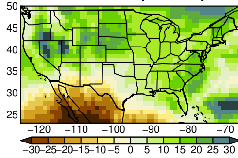
MPI-ESM1-2-HR pr MAM ssp370
