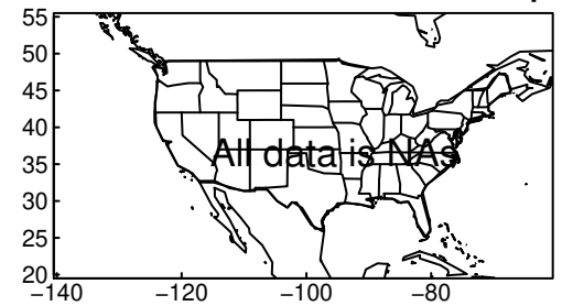
HadGEM3-GC31-MM tasmax SON ssp5
