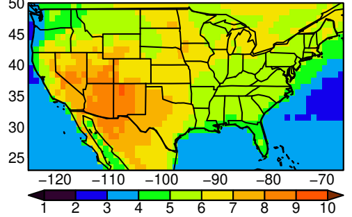
CNRM-CM6-1-HR tasmax JJA ssp58
