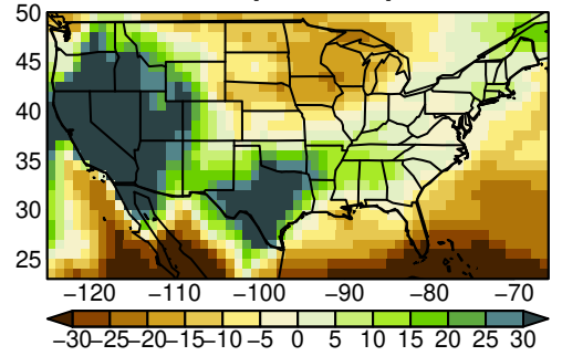
CESM2 pr SON ssp585
