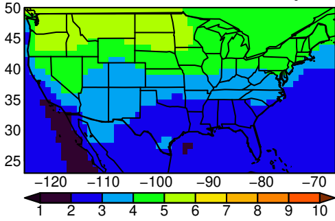
IPSL-CM6A-LR tasmax SON ssp245
