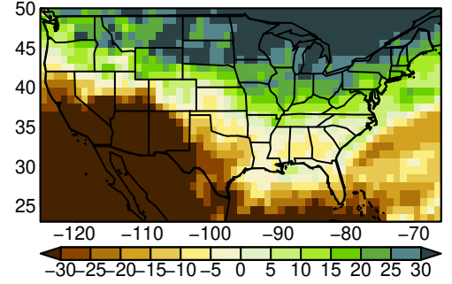
CNRM-CM6-1-HR pr JJA ssp585
