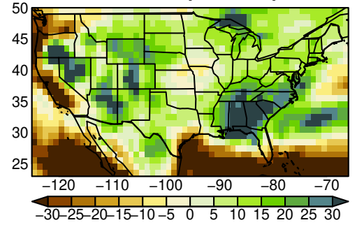
MRI-ESM2-0 pr SON ssp585
