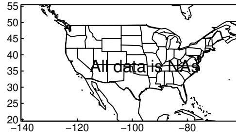
HadGEM3-GC31-MM tasmax MAM ssp3
