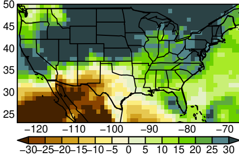
EC-Earth3 pr MAM ssp370
