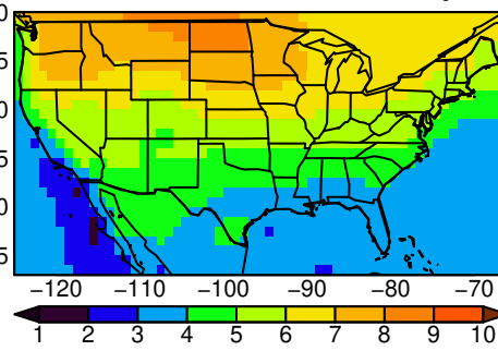
IPSL-CM6A-LR tasmax SON ssp370
