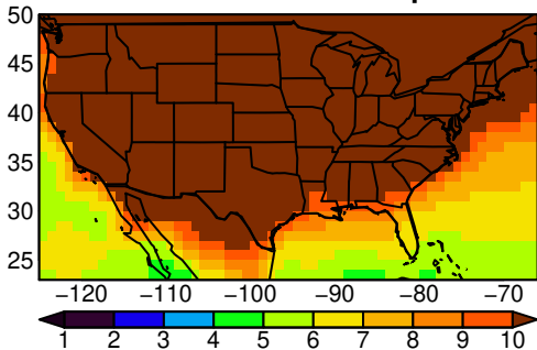
NESM3 tasmax SON ssp245
