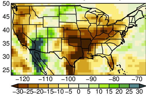
BCC-CSM2-MR pr SON ssp245
