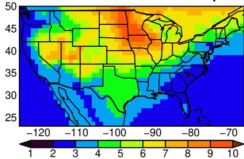
CNRM-ESM2-1 tasmin MAM ssp370
