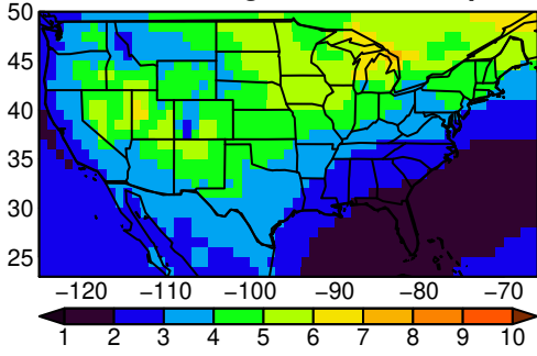
EC-Earth3-Veg tasmin MAM ssp245
