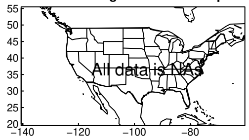
EC-Earth3-Veg tasmax SON ssp585
