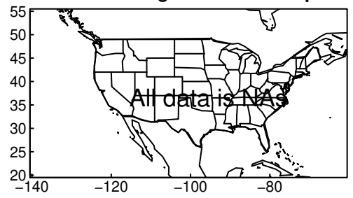
EC-Earth3-Veg tasmax DJF ssp585
