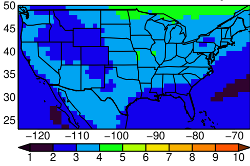
IPSL-CM6A-LR tasmax MAM ssp245
