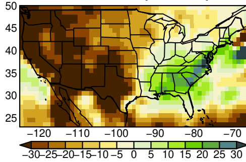
MPI-ESM1-2-LR pr SON ssp370
