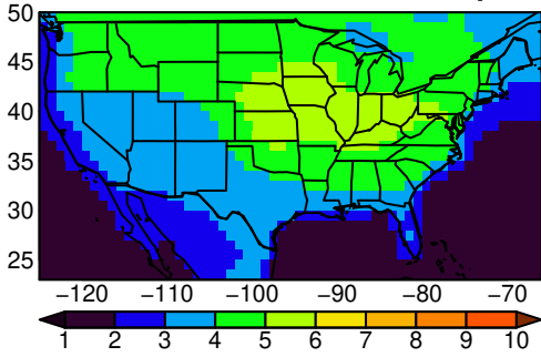
BCC-CSM2-MR tasmax SON ssp245
