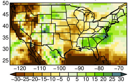
EC-Earth3 pr SON ssp585
