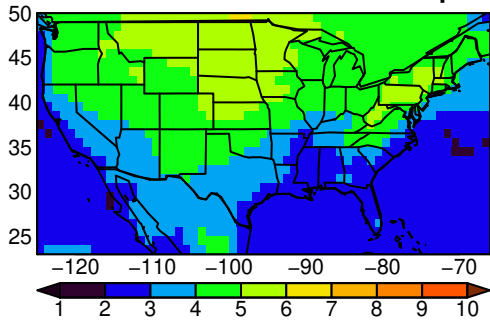
MPI-ESM1-2-HR tasmax SON ssp37i
