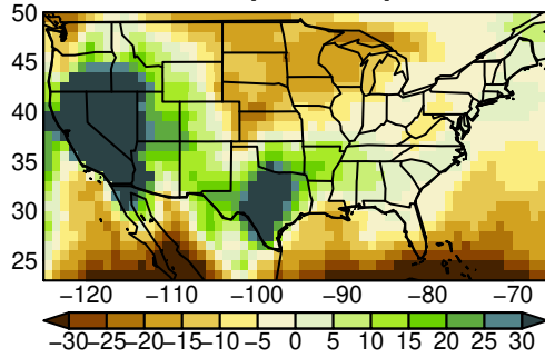
CESM2 pr SON ssp370
