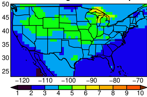
EC-Earth3-Veg tasmax SON ssp245
