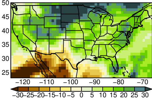
EC-Earth3 pr MAM ssp245
