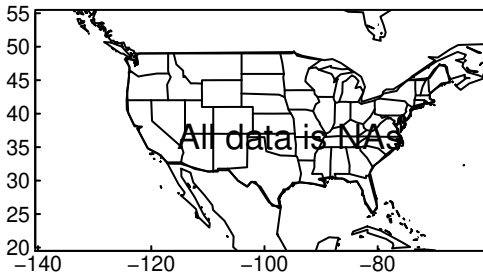
NESM3 tasmin SON ssp370
