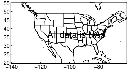
GISS-E2-1-G tasmin DJF ssp585
