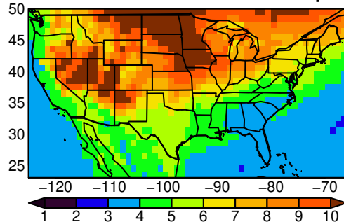
CNRM-CM6-1-HR tasmin MAM ssp58
