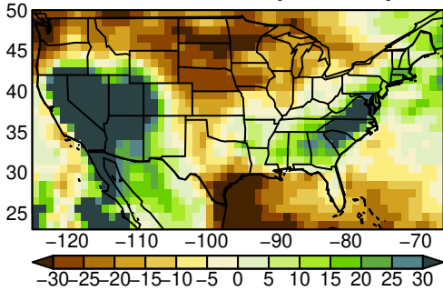
HadGEM3-GC31-LL pr SON ssp245
