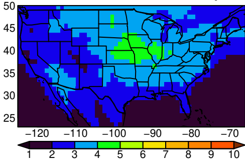
BCC-CSM2-MR tasmin SON ssp245
