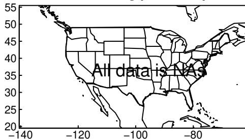
EC-Earth3-Veg pr DJF ssp585
