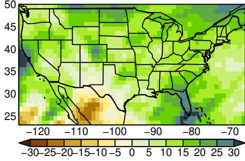
BCC-CSM2-MR pr MAM ssp245
