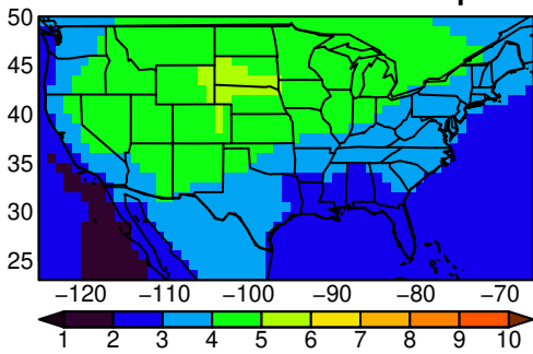
CNRM-CM6-1 tasmx SON ssp245
