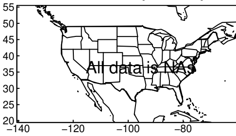
CNRM-CM6-1-HR pr JJA ssp245
