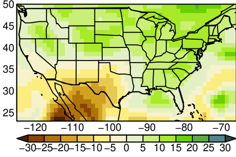
MPI-ESM1-2-LR pr MAM ssp245
