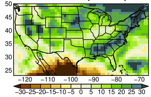
MPI-ESM1-2-HR pr MAM ssp585
