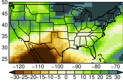
CESM2 pr MAM ssp245
