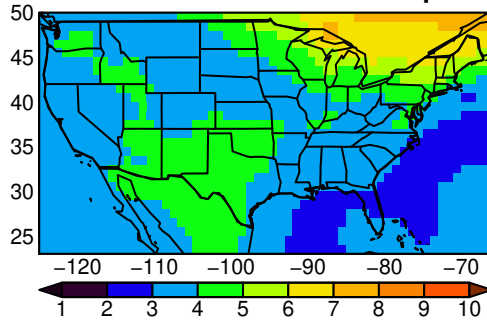
ACCESS-CM2 tasmax MAM ssp370
