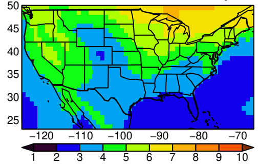
BCC-CSM2-MR tasmax MAM ssp585
