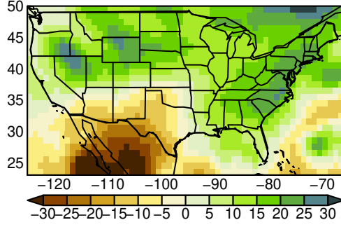
MPI-ESM1-2-LR pr MAM ssp370
