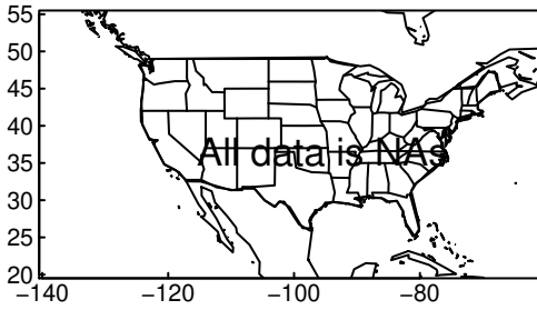
NESM3 tasmin MAM ssp370
