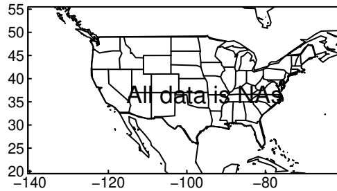
HadGEM3-GC31-LL tasmax SON ssp3
