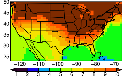
HadGEM3-GC31-LL tasmax SON ssp5
