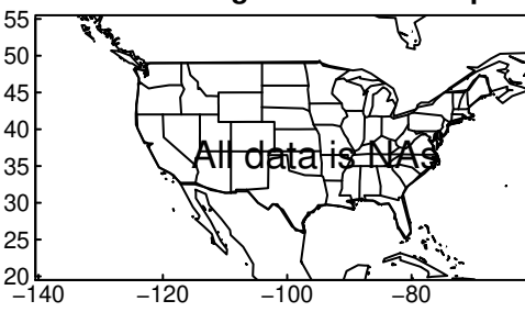
EC-Earth3-Veg tasmax SON ssp370
