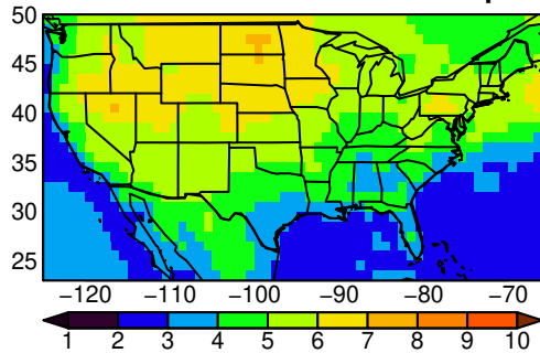
AWI-CM-1-1-MR tasmin SON ssp37f
