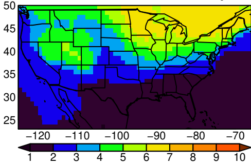
BCC-CSM2-MR tasmin MAM ssp245
