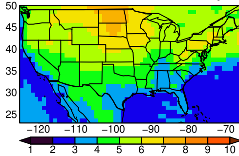
AWI-CM-1-1-MR tasmax SON ssp37i
