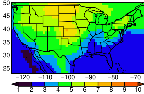
MPI-ESM1-2-LR tasmax SON ssp37f
