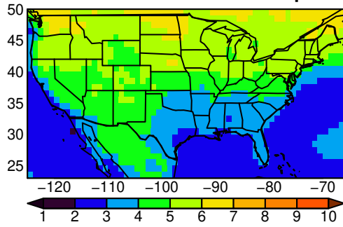
NorESM2-MM tasmx SON ssp370
