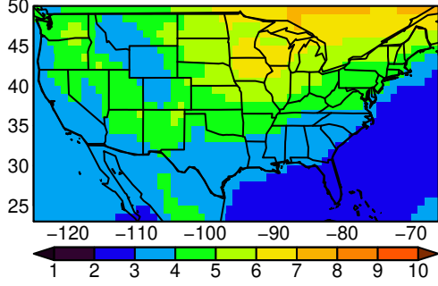
HadGEM3-GC31-LL tasmax MAM ssp2
