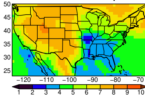
NESM3 tasmax SON ssp585
