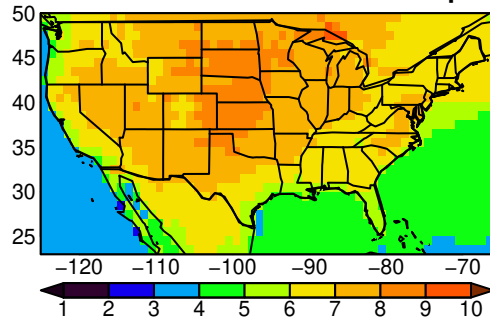
CNRM-CM6-1-HR tasmin SON ssp58
