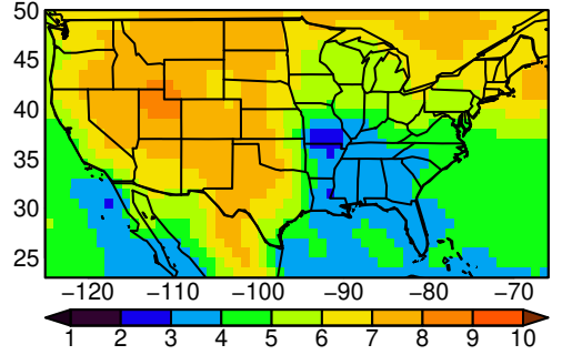
NESM3 tasmin SON ssp585
