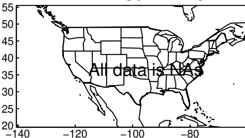
EC-Earth3-Veg pr DJF ssp370
