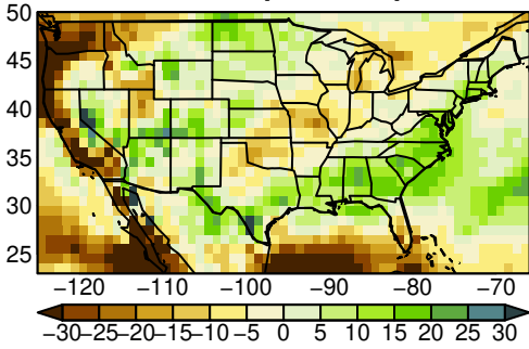
EC-Earth3 pr SON ssp245
