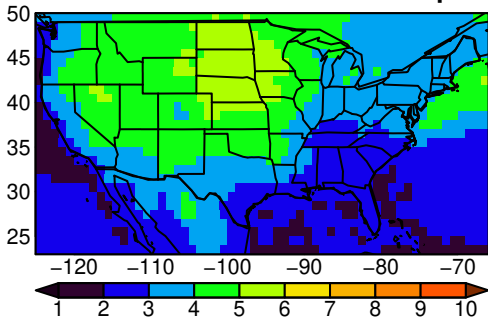
AWI-CM-1-1-MR tasmin SON ssp24f
