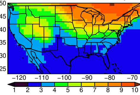
BCC-CSM2-MR tasmin MAM ssp370
