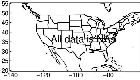
NorCPM1 pr MAM ssp245
