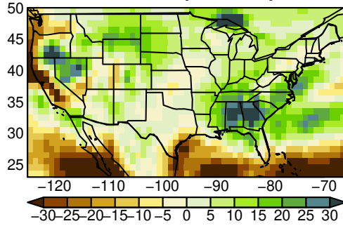
MRI-ESM2-0 pr SON ssp370
