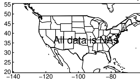
HadGEM3-GC31-MM tasmax SON ssp5
