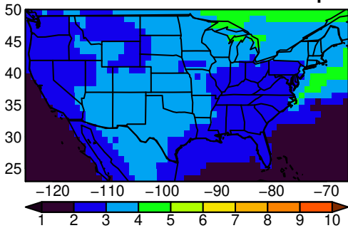
AWI-CM-1-1-MR tasmin JJA ssp24f
