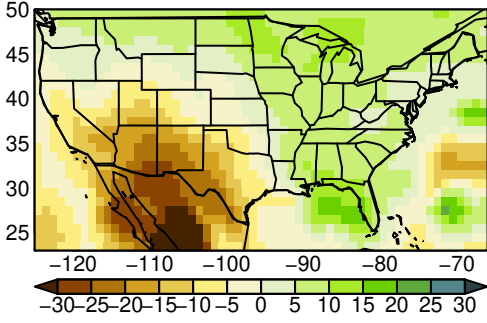
MPI-ESM1-2-LR pr JJA ssp245
