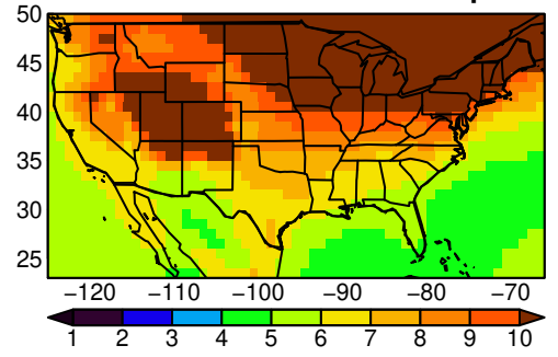
UKESM1-0-LL tasmin MAM ssp585
