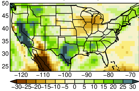
CESM2 pr SON ssp245
