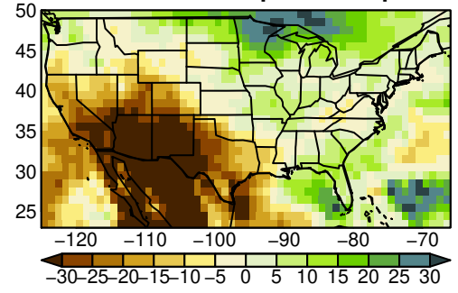
MPI-ESM1-2-HR pr JJA ssp585
