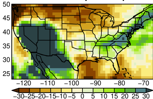
UKESM1-0-LL pr SON ssp245
