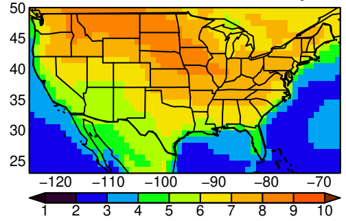
BCC-CSM2-MR tasmax SON ssp585
