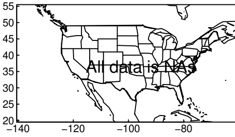
HadGEM3-GC31-LL pr MAM ssp370
