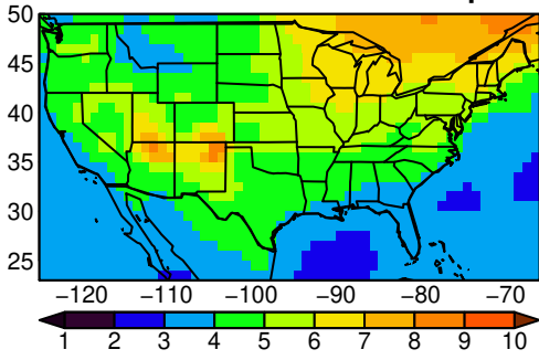
UKESM1-0-LL tasmax MAM ssp245
