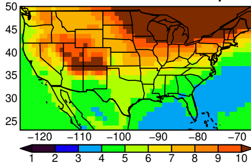
UKESM1-0-LL tasmin MAM ssp370
