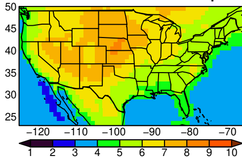
CNRM-ESM2-1 tasmin SON ssp585
