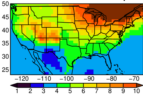
UKESM1-0-LL tasmin MAM ssp245
