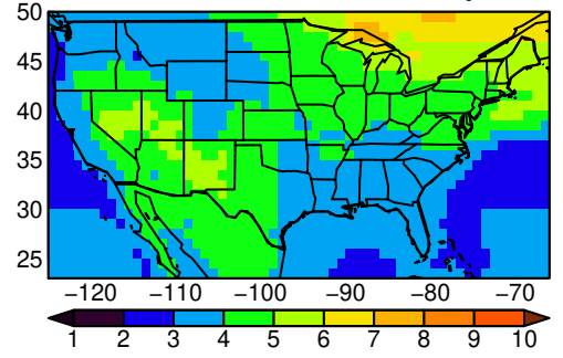
MRI-ESM2-0 tasmax MAM ssp585
