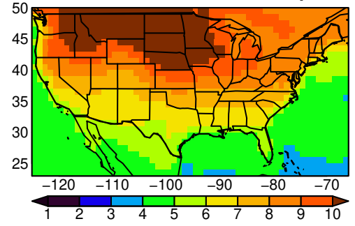
ACCESS-CM2 tasmax SON ssp585
