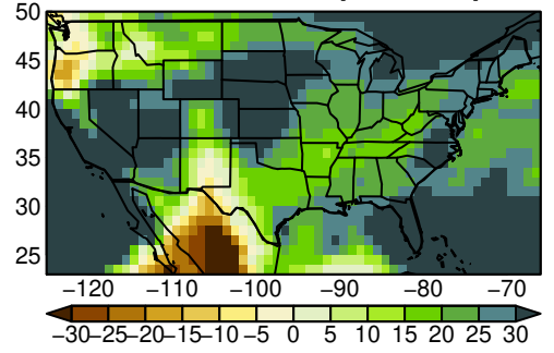
HadGEM3-GC31-LL pr MAM ssp585
