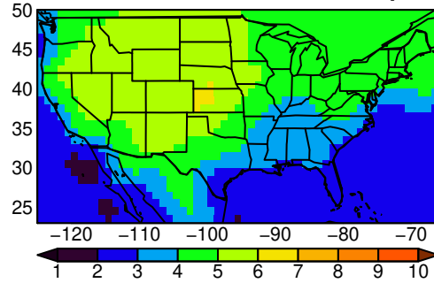
MPI-ESM1-2-LR tasmin SON ssp370
