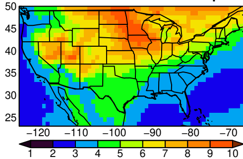
CNRM-ESM2-1 tasmin MAM ssp585
