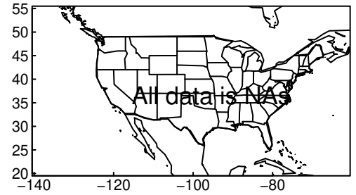
MPI-ESM1-2-LR tasmin DJF ssp585
