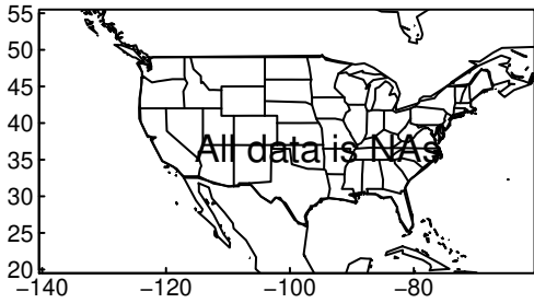
HadGEM3-GC31-MM pr DJF ssp245
