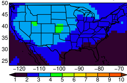
MPI-ESM1-2-LR tasmin SON ssp245
