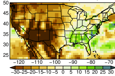
MPI-ESM1-2-HR pr SON ssp370
