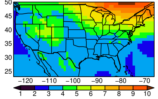
MRI-ESM2-0 tasmin MAM ssp585
