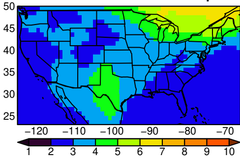
ACCESS-CM2 tasmax MAM ssp245
