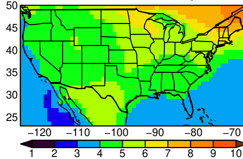
NESM3 tasmax MAM ssp585
