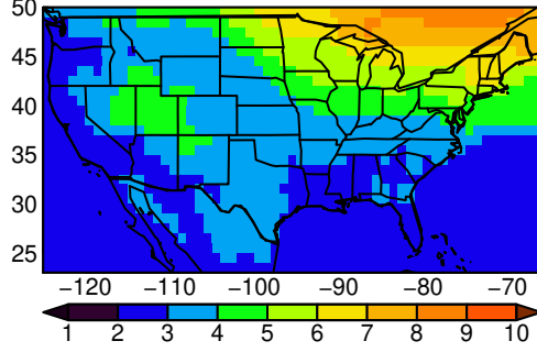
MRI-ESM2-0 tasmin MAM ssp370
