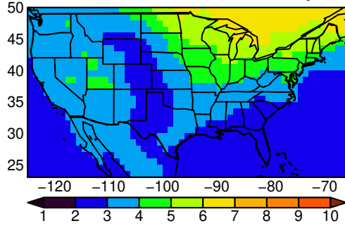
BCC-CSM2-MR tasmax MAM ssp370
