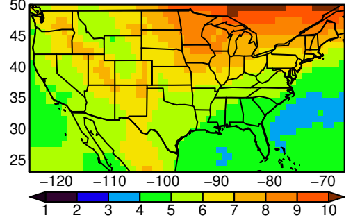
HadGEM3-GC31-LL tasmax MAM ssp5
