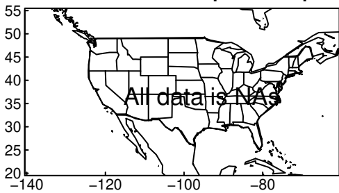
HadGEM3-GC31-MM pr SON ssp245
