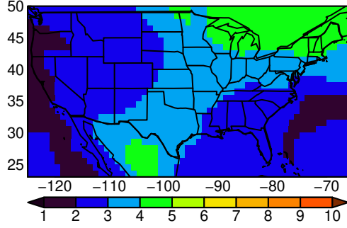
MPI-ESM1-2-LR tasmax MAM ssp37f
