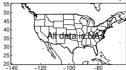
HadGEM3-GC31-MM tasmin DJF ssp2
