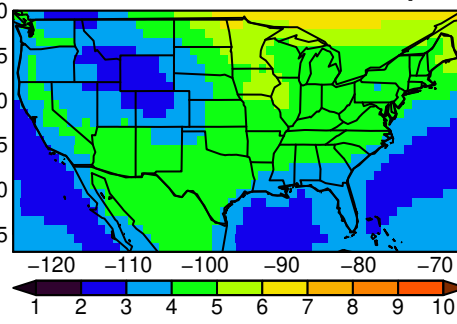
IPSL-CM6A-LR tasmax MAM ssp370
