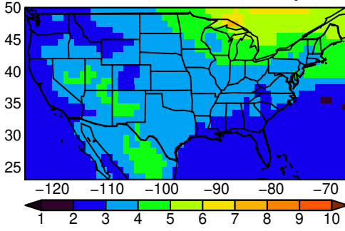
MRI-ESM2-0 tasmax MAM ssp370
