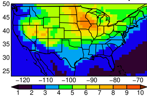
CNRM-ESM2-1 tasmin MAM ssp245
