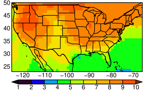
HadGEM3-GC31-LL tasmin SON ssp5
