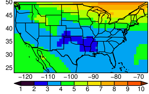
ACCESS-ESM1-5 tasmin MAM ssp58i
