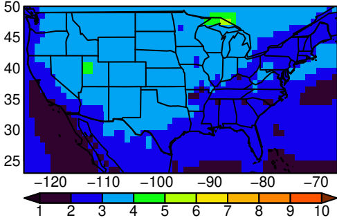
MRI-ESM2-0 tasmin SON ssp245
