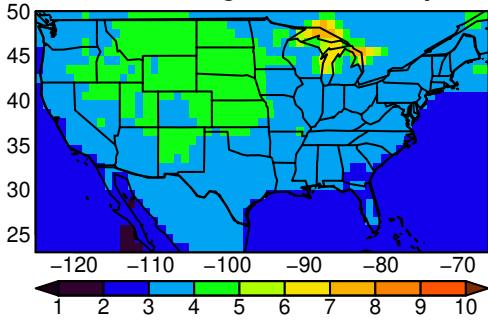
EC-Earth3-Veg tasmin SON ssp245
