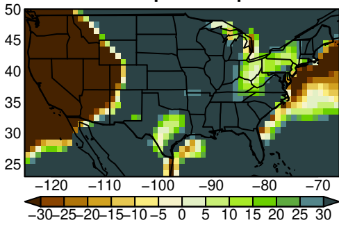
NESM3 pr SON ssp245
