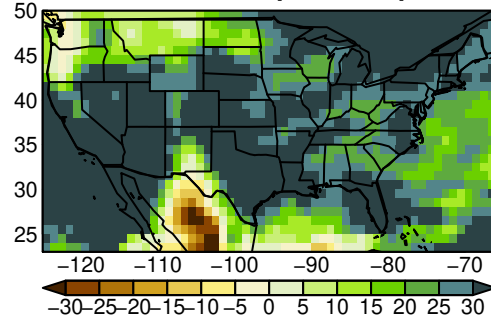
UKESM1-0-LL pr MAM ssp585
