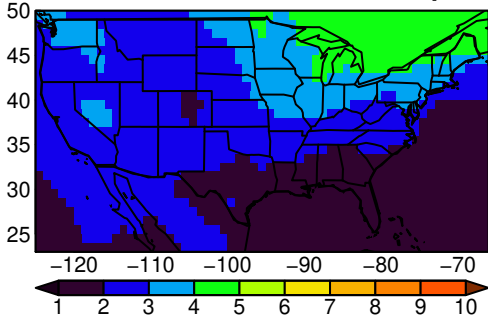
BCC-CSM2-MR tasmax MAM ssp245
