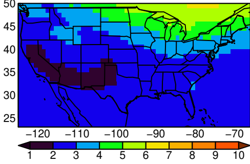
ACCESS-ESM1-5 tasmin MAM ssp24i
