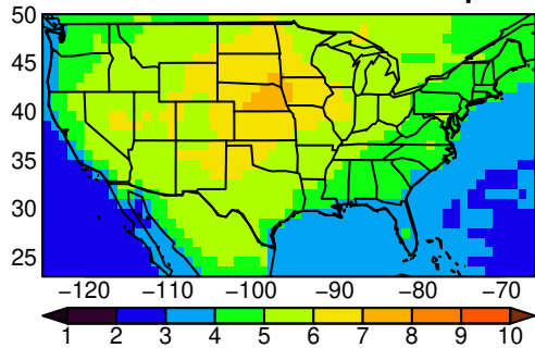
CNRM-ESM2-1 tasmin SON ssp370
