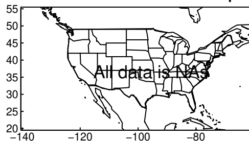
AWI-CM-1-1-MR tasmin SON ssp58f
