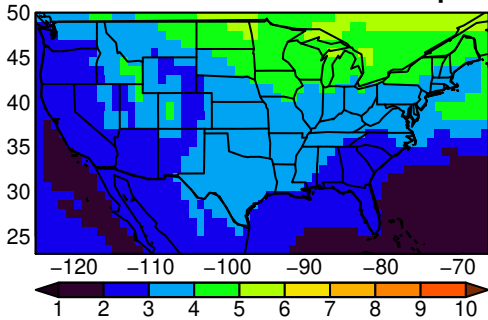
AWI-CM-1-1-MR tasmin MAM ssp24f
