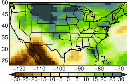
CESM2 pr JJA ssp245
