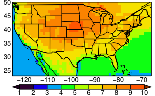
CNRM-CM6-1-HR tasmax SON ssp58
