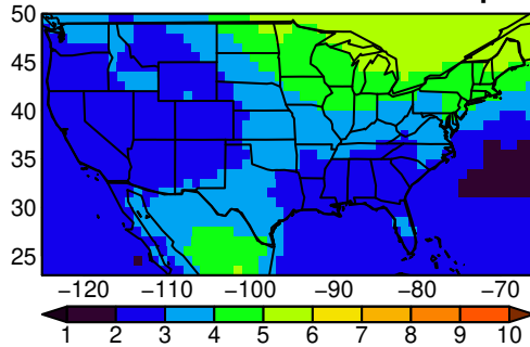
MPI-ESM1-2-HR tasmax MAM ssp58i
