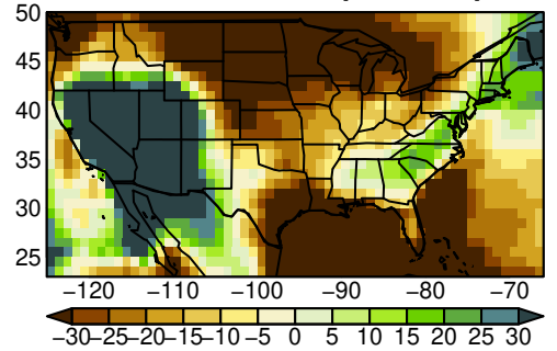
HadGEM3-GC31-LL pr SON ssp585
