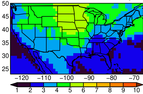
AWI-CM-1-1-MR tasmax SON ssp24i
