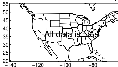
HadGEM3-GC31-MM tasmin MAM ssp3
