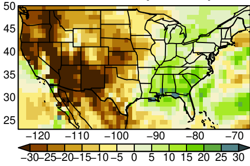
MPI-ESM1-2-HR pr SON ssp245
