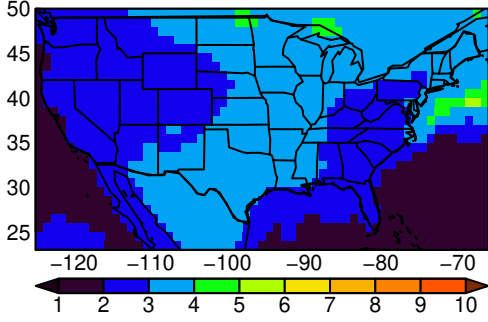
AWI-CM-1-1-MR tasmax MAM ssp24i
