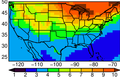
HadGEM3-GC31-LL tasmin MAM ssp2
