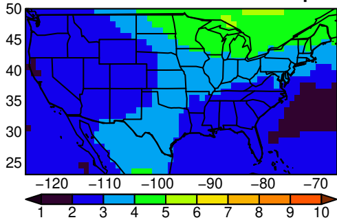
MPI-ESM1-2-HR tasmax MAM ssp37i
