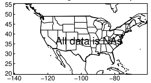
EC-Earth3-Veg tasmin SON ssp585
