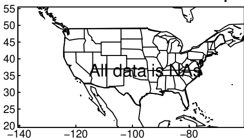
CNRM-CM6-1-HR tasmin SON ssp24
