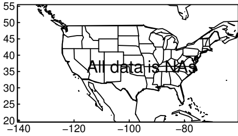
HadGEM3-GC31-MM pr MAM ssp245
