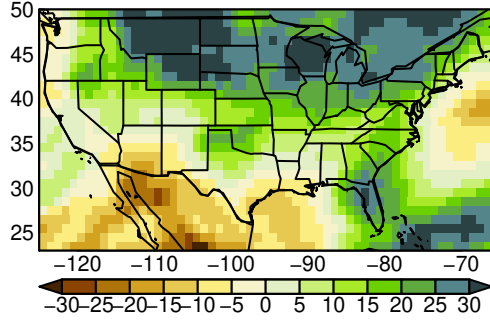
CESM2 pr JJA ssp370
