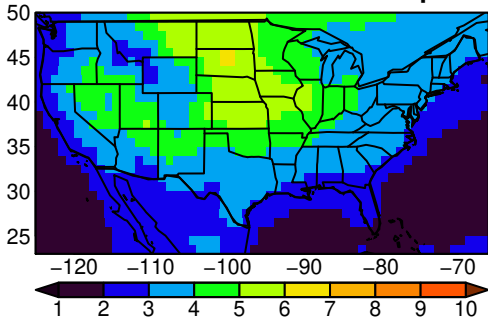
CNRM-CM6-1 tasmx MAM ssp245
