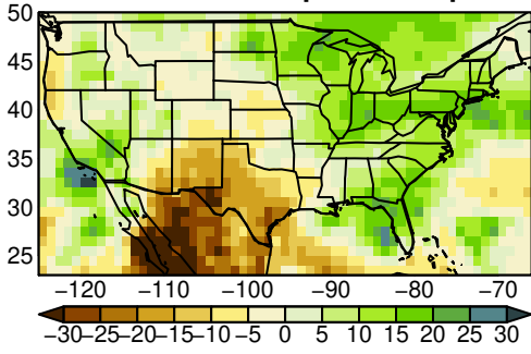
MPI-ESM1-2-HR pr JJA ssp245
