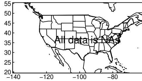
HadGEM3-GC31-MM tasmax DJF ssp3
