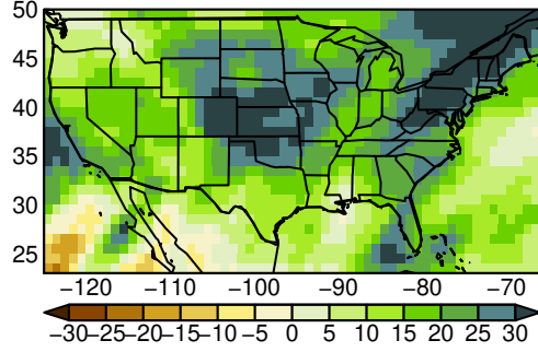
BCC-CSM2-MR pr MAM ssp370
