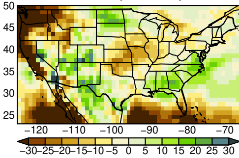
EC-Earth3 pr SON ssp370
