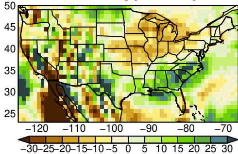
EC-Earth3-Veg pr SON ssp245
