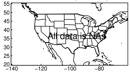
MPI-ESM1-2-LR pr JJA ssp585
