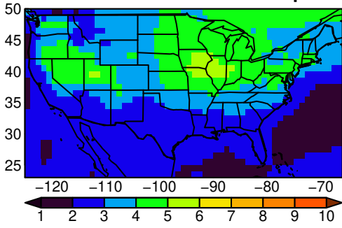
NorESM2-MM tasmx MAM ssp245
