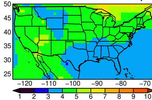
ACCESS-ESM1-5 tasmax MAM ssp58
