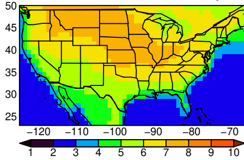
BCC-CSM2-MR tasmax SON ssp370
