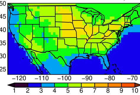
BCC-CSM2-MR tasmin SON ssp370
