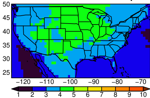
CNRM-ESM2-1 tasmin SON ssp245
