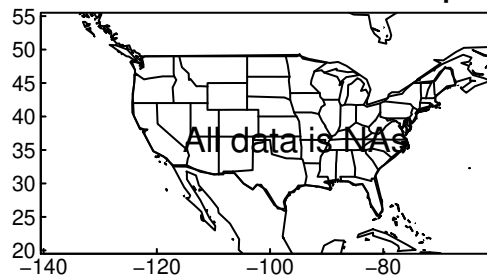
AWI-CM-1-1-MR tasmin DJF ssp58f
