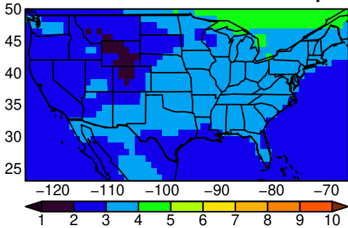
ACCESS-ESM1-5 tasmax MAM ssp24
