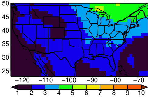
MRI-ESM2-0 tasmax MAM ssp245
