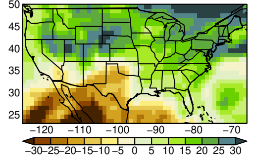
MRI-ESM2-0 pr MAM ssp585
