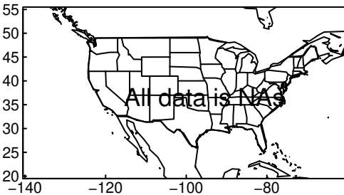
EC-Earth3-Veg pr SON ssp370
