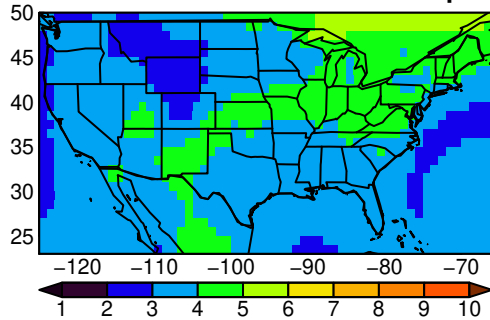
ACCESS-ESM1-5 tasmax MAM ssp37
