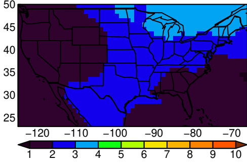
MPI-ESM1-2-LR tasmax MAM ssp24f
