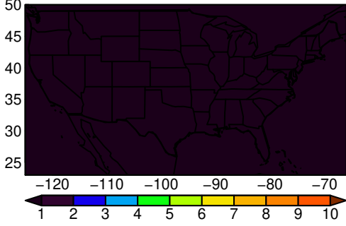
NESM3 tasmin MAM ssp245
