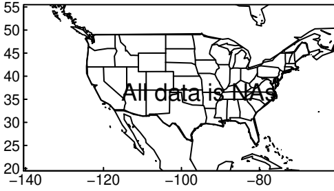
CNRM-CM6-1-HR tasmax DJF ssp37
