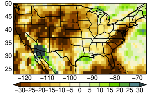
CNRM-CM6-1-HR pr SON ssp585
