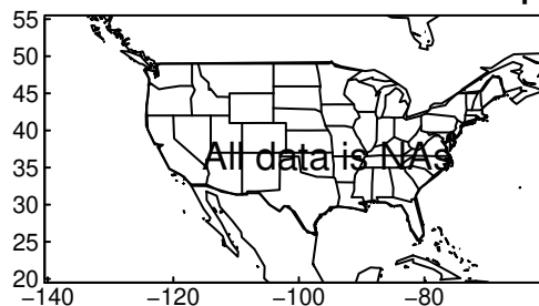
HadGEM3-GC31-MM tasmin SON ssp3
