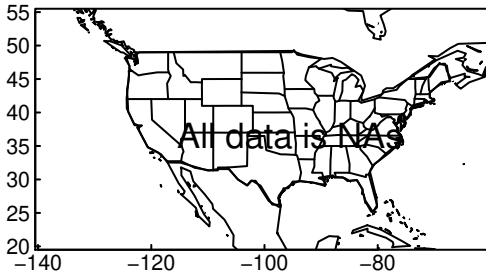
NorCPM1 pr DJF ssp370
