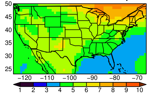
ACCESS-CM2 tasmax MAM ssp585
