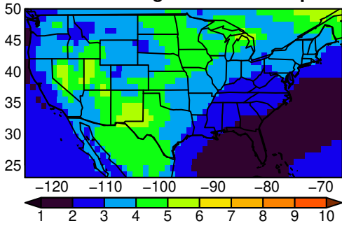
EC-Earth3-Veg tasmax MAM ssp245
