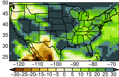
UKESM1-0-LL pr MAM ssp370
