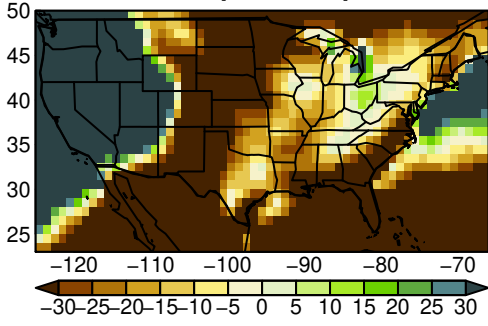
NESM3 pr MAM ssp245
