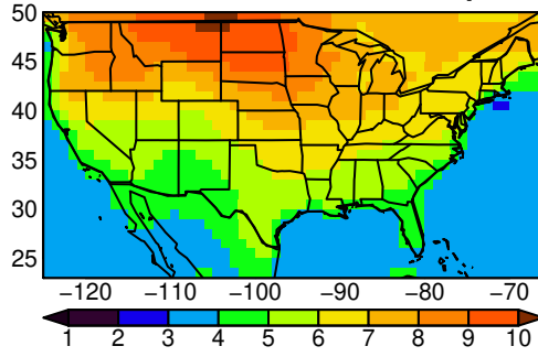
ACCESS-CM2 tasmax SON ssp370
