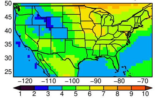
IPSL-CM6A-LR tasmax MAM ssp585
