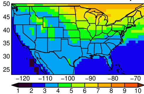
AWI-CM-1-1-MR tasmin MAM ssp37f
