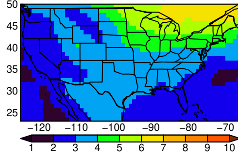
MPI-ESM1-2-LR tasmin MAM ssp370
