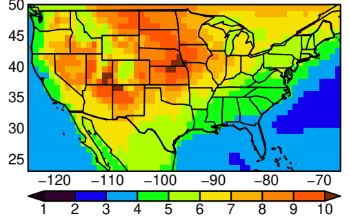
CNRM-CM6-1-HR tasmax MAM ssp58
