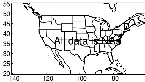
HadGEM3-GC31-LL tasmin SON ssp3
