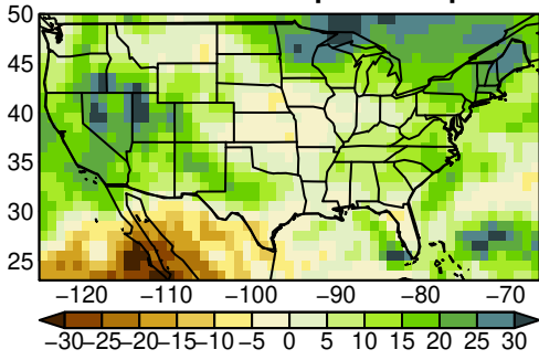
MPI-ESM1-2-HR pr MAM ssp245
