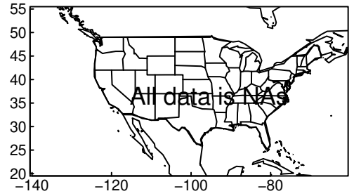
MPI-ESM1-2-LR pr MAM ssp585
