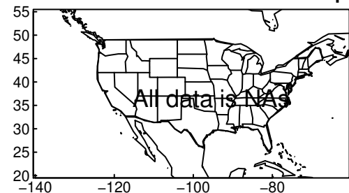
HadGEM3-GC31-MM tasmin MAM ssp1
