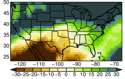
CESM2 pr MAM ssp585
