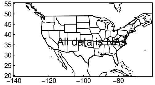
MPI-ESM1-2-LR pr DJF ssp585
