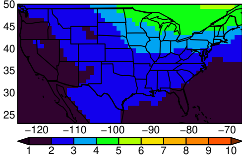
MPI-ESM1-2-LR tasmin MAM ssp245
