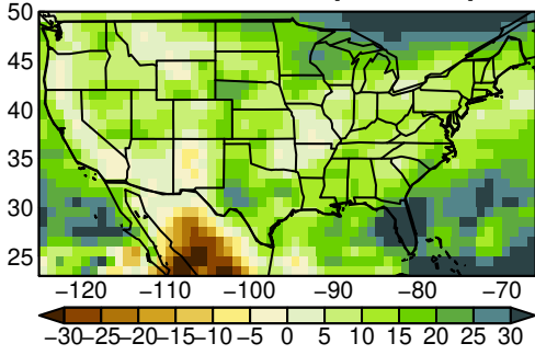
HadGEM3-GC31-LL pr MAM ssp245
