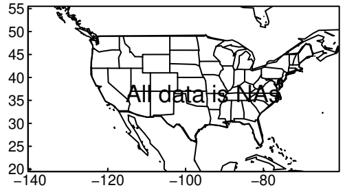
CESM2-FV2 pr JJA ssp585
