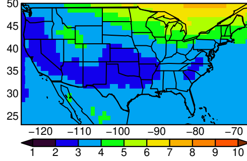
ACCESS-ESM1-5 tasmin MAM ssp37i
