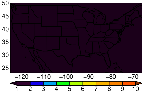
NESM3 tasmax MAM ssp245
