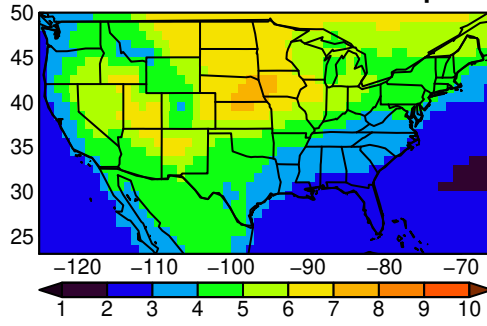
CNRM-CM6-1 tasmx MAM ssp370
