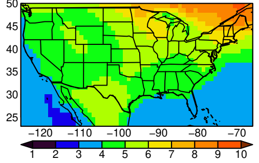
NESM3 tasmin MAM ssp585
