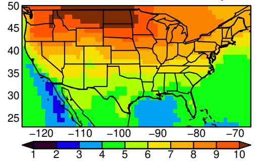
IPSL-CM6A-LR tasmax SON ssp585
