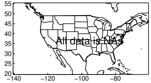
AWI-CM-1-1-MR tasmax MAM ssp58i
