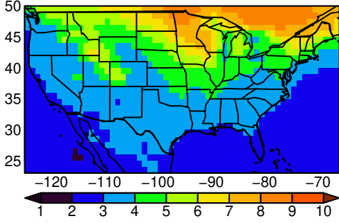
IPSL-CM6A-LR tasmin MAM ssp245
