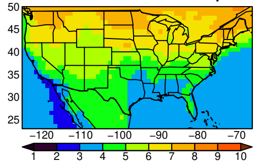
NorESM2-MM tasmx SON ssp585
