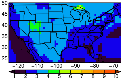
MRI-ESM2-0 tasmax SON ssp245
