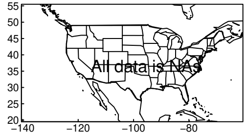
AWI-CM-1-1-MR tasmax DJF ssp58i
