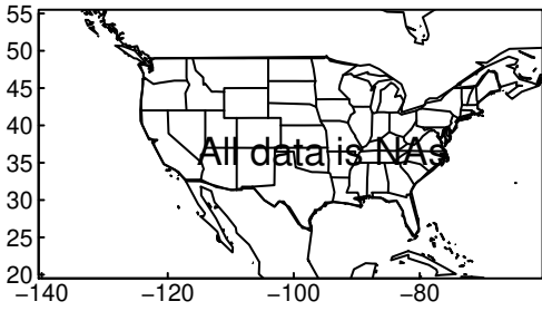
NorCPM1 pr DJF ssp245
