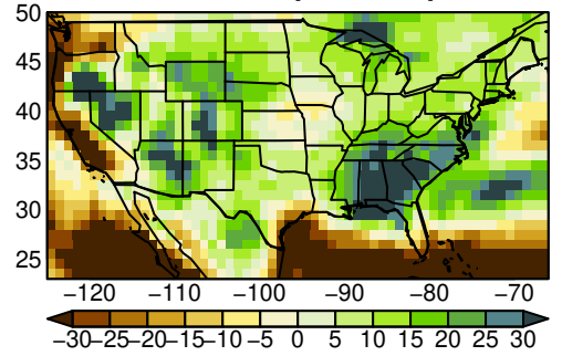
MRI-ESM2-0 pr SON ssp585
