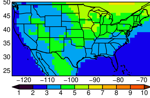
MMEA-MEDIAN tasmx MAM ssp370 n=
