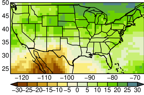
MMEA-MEDIAN pr MAM ssp245 n= 2
