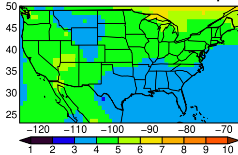
ACCESS-ESM1-5 tasmax MAM ssp58
