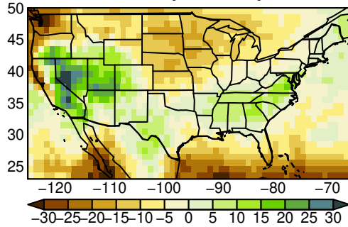
MMEA-MEDIAN pr SON ssp370 n= 1
