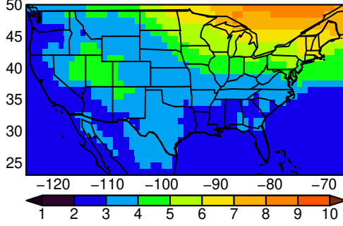
MRI-ESM2-0 tasmin MAM ssp370
