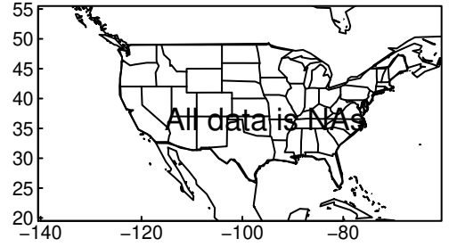
TaiESM1 tasmin DJF ssp585
