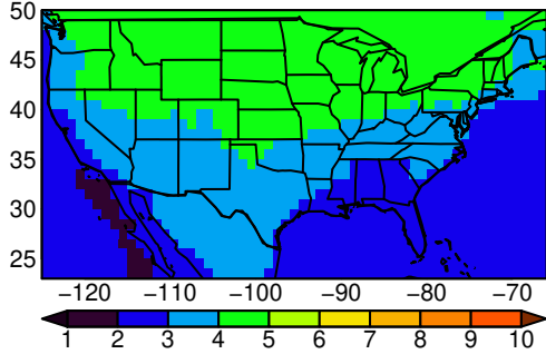
MMEA-MEDIAN tasmx SON ssp245 n=
