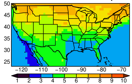
NorESM2-MM tasmax SON ssp585
