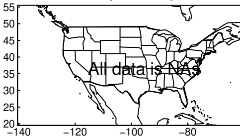
NESM3 pr DJF ssp370
