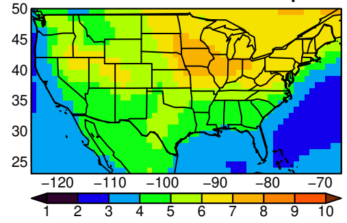
NorESM2-LM tasmx MAM ssp585
