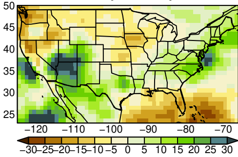
MIROC6 pr SON ssp245
