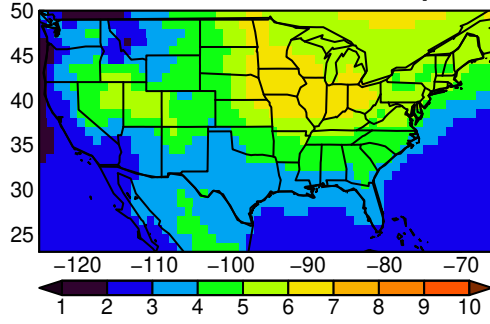
NorESM2-MM tasmax MAM ssp370
