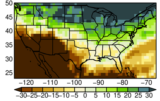
CNRM-CM6-1-HR pr JJA ssp585
