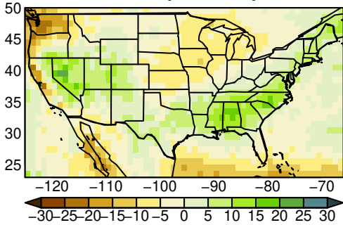
MMEA-MEDIAN pr SON ssp245 n= 2
