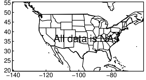
TaiESM1 tasmin MAM ssp585
