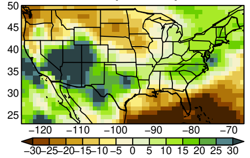
MIROC6 pr SON ssp585
