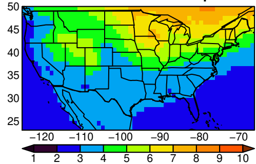
MMEA-MEDIAN tasmin MAM ssp370 n=
