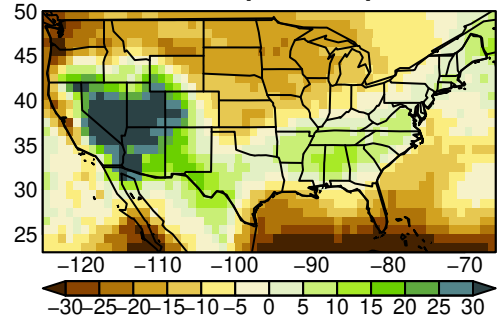
MMEA-MEDIAN pr SON ssp585 n= 1
