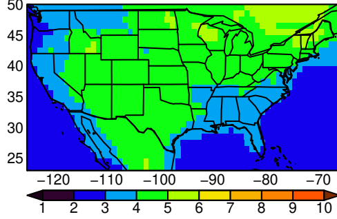
MMEA-MEDIAN tasmx JJA ssp370 n=
