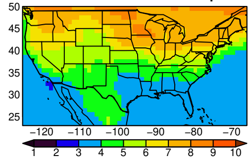
NorESM2-LM tasmx SON ssp585
