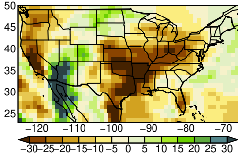
BCC-CSM2-MR pr SON ssp245
