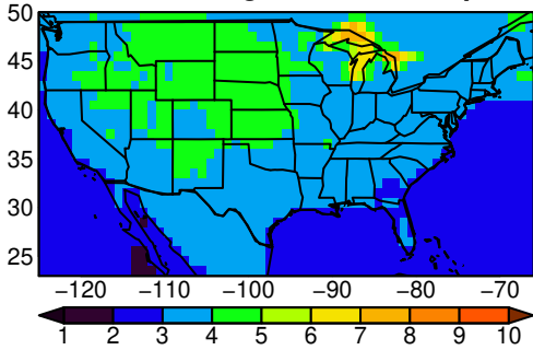
EC-Earth3-Veg tasmin SON ssp245
