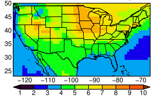
NorESM2-MM tasmax MAM ssp585
