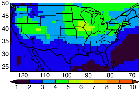
NorESM2-MM tasmax MAM ssp245
