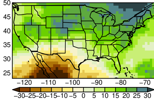
MMEA-MEDIAN pr MAM ssp370 n= 1
