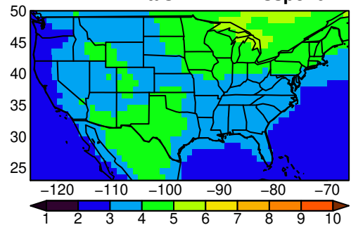
MMEA-MEDIAN tasmin JJA ssp370 n=
