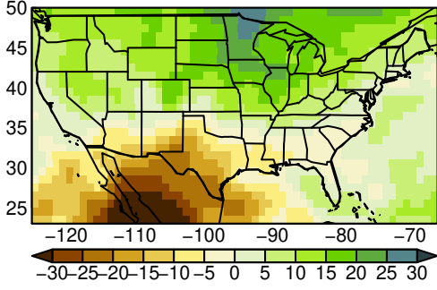
MIROC6 pr MAM ssp245
