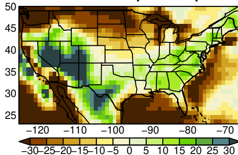
IPSL-CM6A-LR pr SON ssp585
