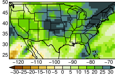
BCC-CSM2-MR pr MAM ssp370
