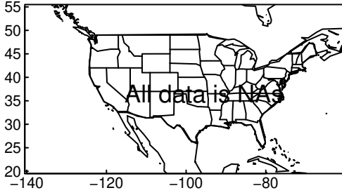
TaiESM1 tasmin MAM ssp370
