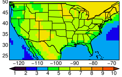
MMEA-MEDIAN tasmx JJA ssp585 n=
