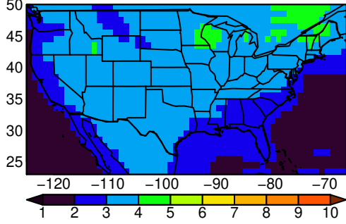
MMEA-MEDIAN tasmx JJA ssp245 n=
