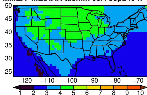
MMEA-MEDIAN tasmin SON ssp245 n=
