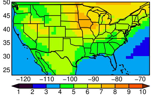
MMEA-MEDIAN tasmx MAM ssp585 n=
