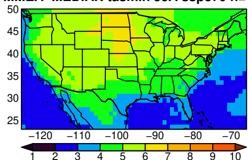
MMEA-MEDIAN tasmin SON ssp370 n=
