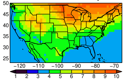
MMEA-MEDIAN tasmin MAM ssp585 n=
