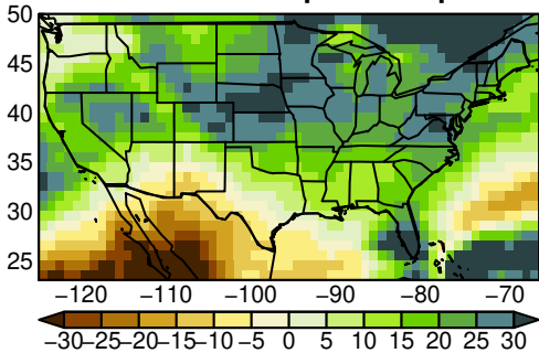
IPSL-CM6A-LR pr MAM ssp370
