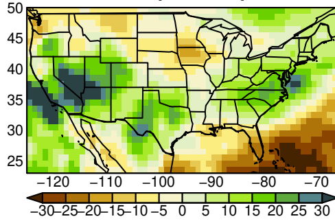
MIROC6 pr SON ssp370
