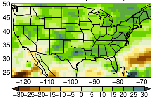
IPSL-CM6A-LR pr MAM ssp245
