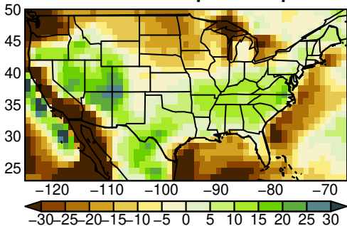
IPSL-CM6A-LR pr SON ssp370
