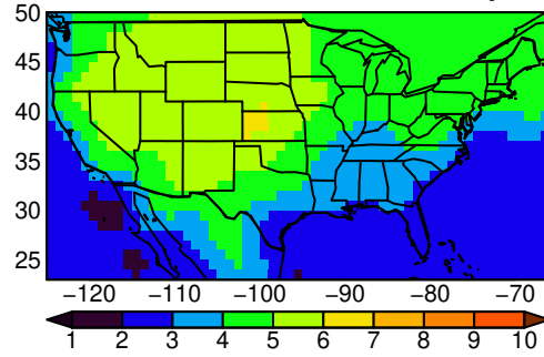
MPI-ESM1-2-LR tasmin SON ssp370
