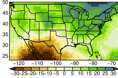
MIROC6 pr MAM ssp370
