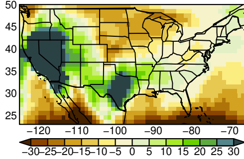
CESM2 pr SON ssp370
