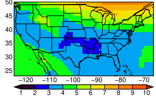
ACCESS-ESM1-5 tasmin MAM ssp58i
