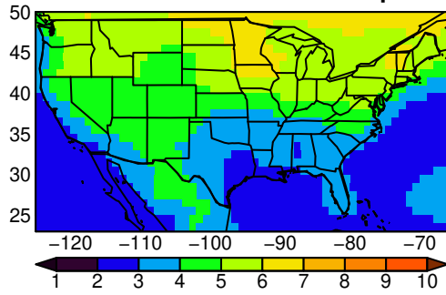
NorESM2-LM tasmx SON ssp370
