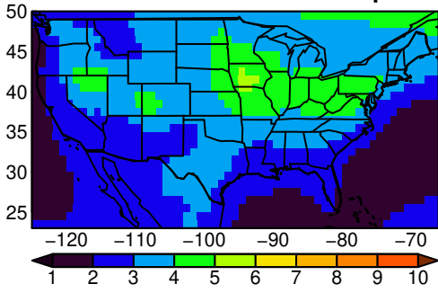
NorESM2-LM tasmx MAM ssp245
