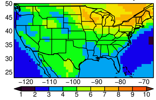
NorESM2-LM tasmx JJA ssp585
