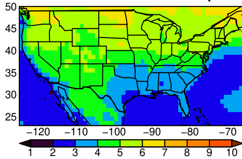
NorESM2-MM tasmax SON ssp370
