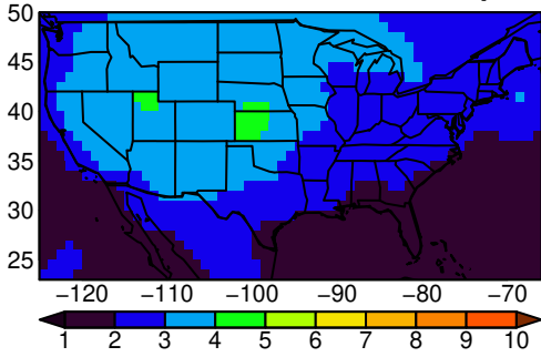
MPI-ESM1-2-LR tasmin SON ssp245
