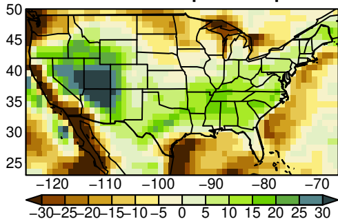
IPSL-CM6A-LR pr SON ssp245
