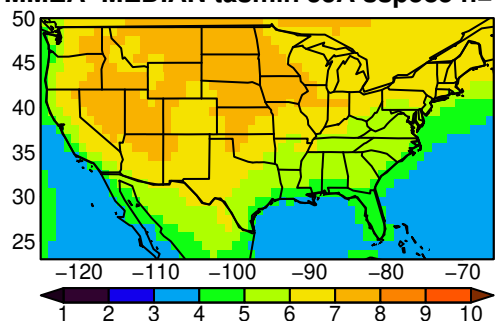
MMEA-MEDIAN tasmin SON ssp585 n=
