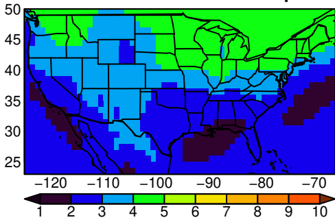
NorESM2-LM tasmx SON ssp245
