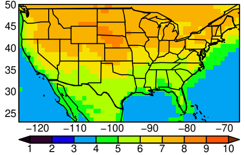
MMEA-MEDIAN tasmx SON ssp585 n=
