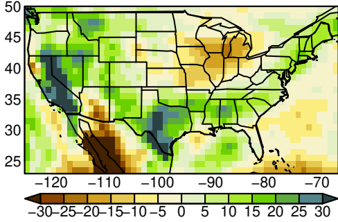
CESM2 pr SON ssp245
