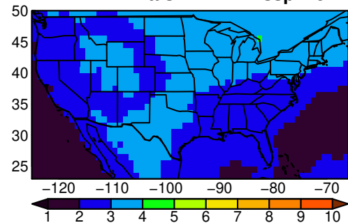
MMEA-MEDIAN tasmin JJA ssp245 n=
