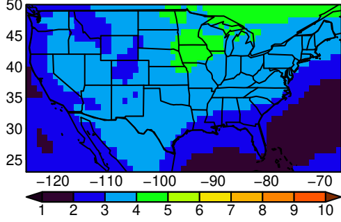
MMEA-MEDIAN tasmx MAM ssp245 n=
