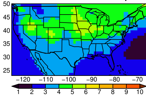
NorESM2-LM tasmx MAM ssp370
