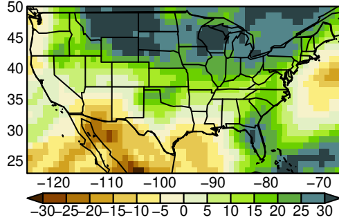
CESM2 pr JJA ssp370
