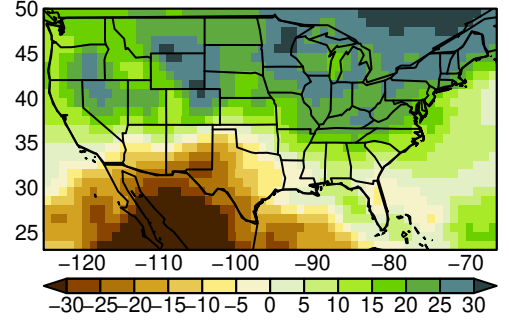
MIROC6 pr MAM ssp585
