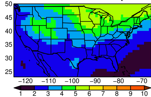
MMEA-MEDIAN tasmin MAM ssp245 n=
