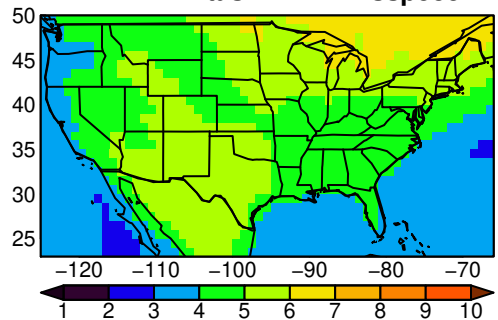
MMEA-MEDIAN tasmin JJA ssp585 n=
