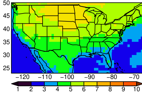
MMEA-MEDIAN tasmx SON ssp370 n=
