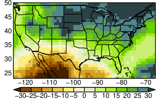
MMEA-MEDIAN pr MAM ssp585 n= 1
